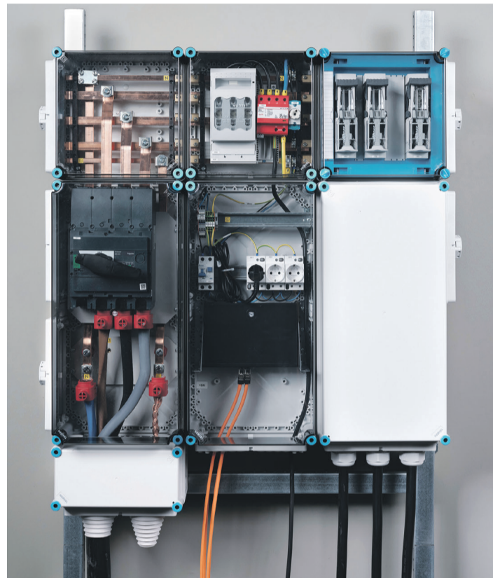
ENYCHARGE Mi EV 44 kW 3001 für Doppelladepunkte mit 22kW Ladeleistung je Ladepunkt. (Bildquelle: Gustav Hensel GmbH & Co. KG)
